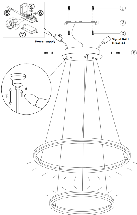
Collegamento - wiring - Câblage Verkabelung - Cableado - Fiação
