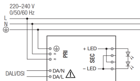
Collegamento - wiring - Câblage Verkabelung - Cableado - Fiação
