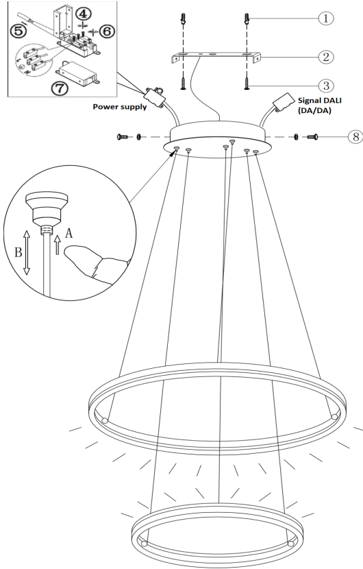
Collegamento - wiring - Câblage Verkabelung - Cableado - Fiação
