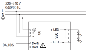
Collegamento - wiring - Câblage Verkabelung - Cableado - Fiação
