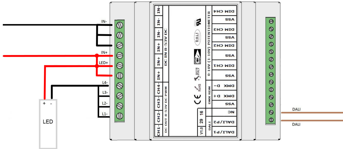
COLLEGAMENTO DALI L406MA02T4A01 - FIGURA N. 7
