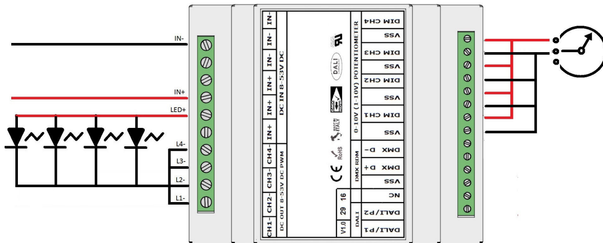
COLLEGAMENTO POTENZIOMETRO MONOCANALE L406MA02T4A01 - FIGURA N. 12
