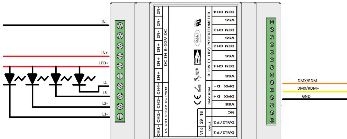
COLLEGAMENTO L406MA02T4A01 A BUS DMX512/RDM - FIGURA N. 2
