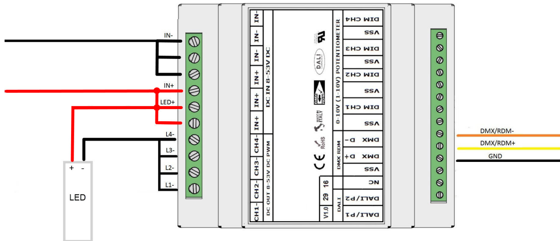
COLLEGAMENTO L406MA02T4A01 A BUS DMX512/RDM - FIGURA N. 4
