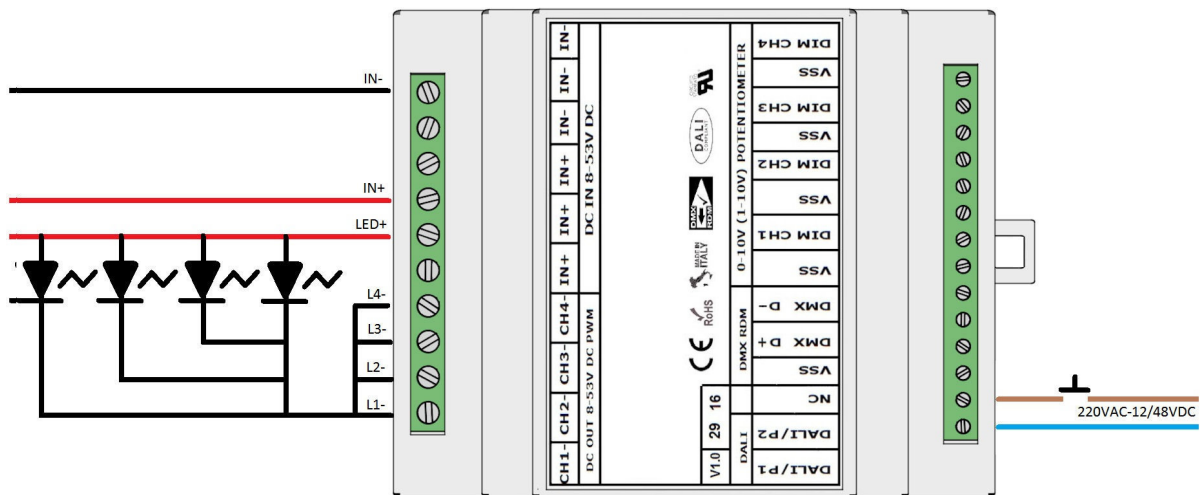
COLLEGAMENTO PULSANTI L406MA02T4A01 - FIGURA N. 9
