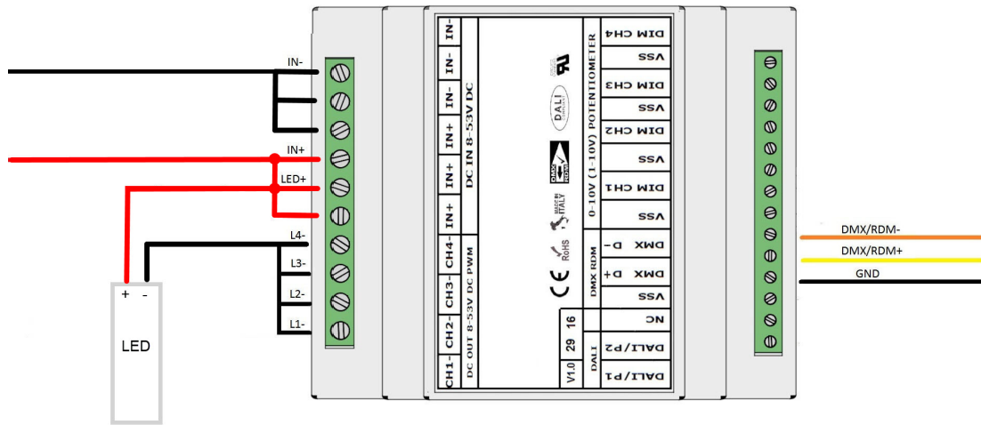
COLLEGAMENTO L406MA02T4A01 A BUS DMX512/RDM - FIGURA N. 5
