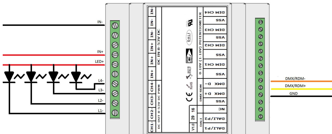
COLLEGAMENTO L406MA02T4A01 A BUS DMX512/RDM - FIGURA N. 3
