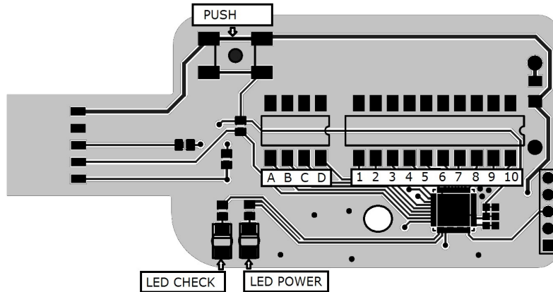
LAYOUT L392MA - FIGURA N. 1
